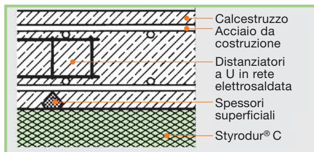
Fig. 19: Spessore superficiale calpestabile in fibrocemento per l'armatura inferiore e intreccio di sostegno in acciaio per l'armatura superiore della soletta.
