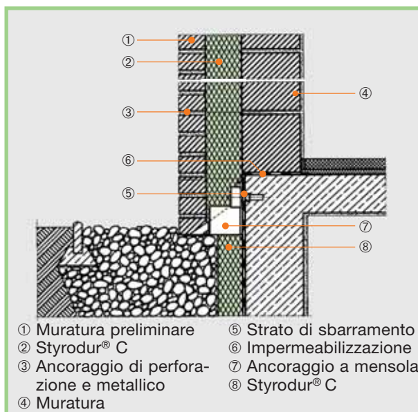
Fig. 31: Collegamento dell'isolamento perimetrale alla muratura con isolamento in intercapedine e ancoraggio a mensola.
