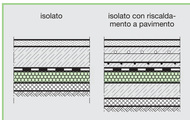
Fig. 22: Strutture del pavimento con Styrodur C.
